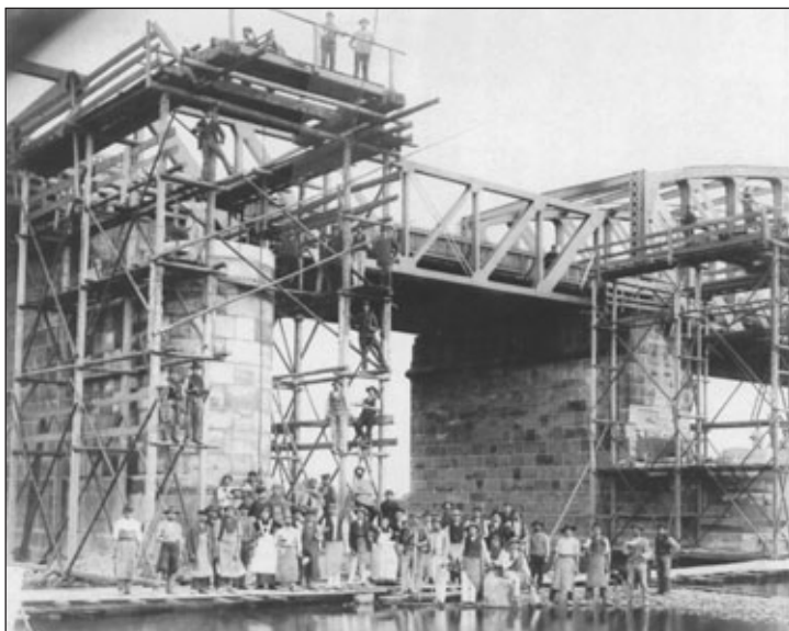
oben: Erweiterungsbau der Brückenpfeiler für das zweite Gleis 1892
