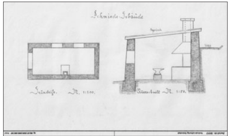
Steinbruch-Schmiedegebäude nach Zeichnung von 1903
