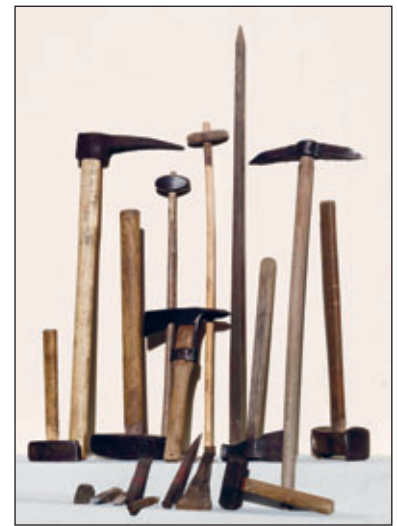
Handwerkzeuge des Steinbruchs
